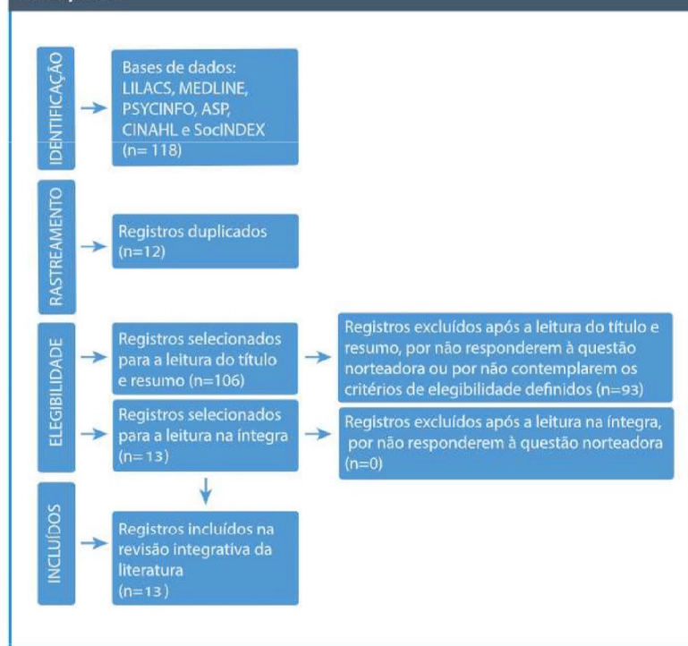
Figura 1. Fluxograma de Estratégia de Busca e Seleção de artigos. Niterói, RJ, Brasil, 2018
